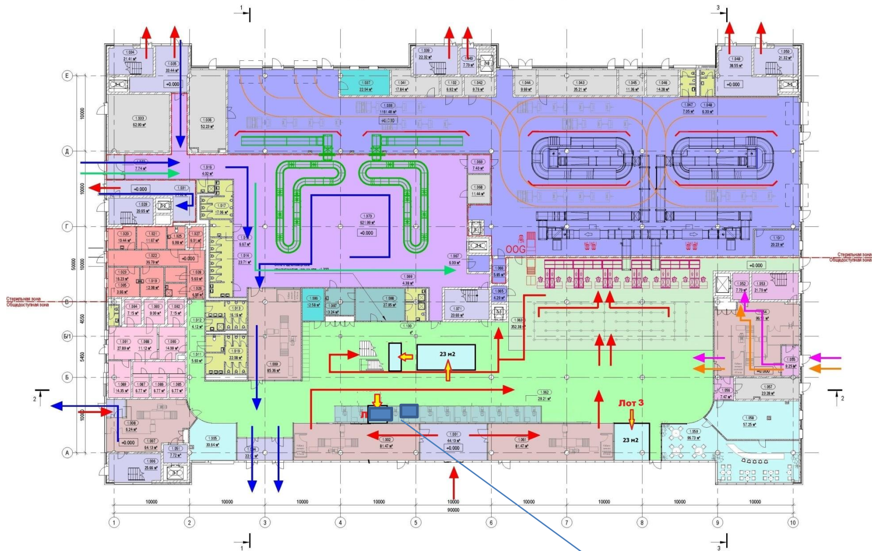
План функционального зонирования 1-го этажа (на отм. 0.000)
